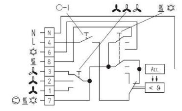
KLR-E 7038 kapcsolási rajza:
